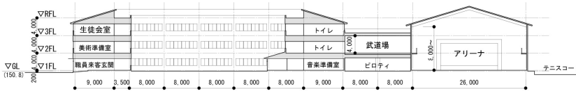
断面図①
