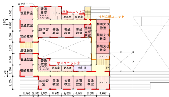
3階平面図
