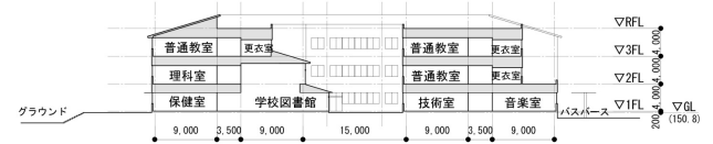
断面図②
