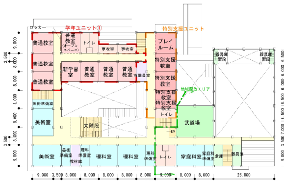
3階平面図
