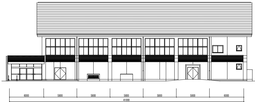
南側立面図
