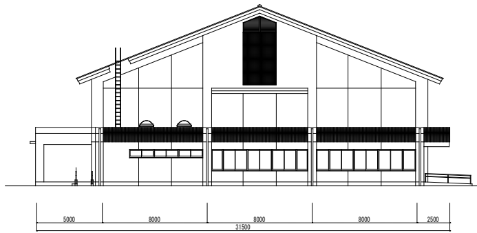
西側立面図
