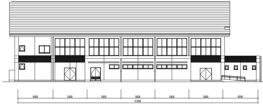
北側立面図
