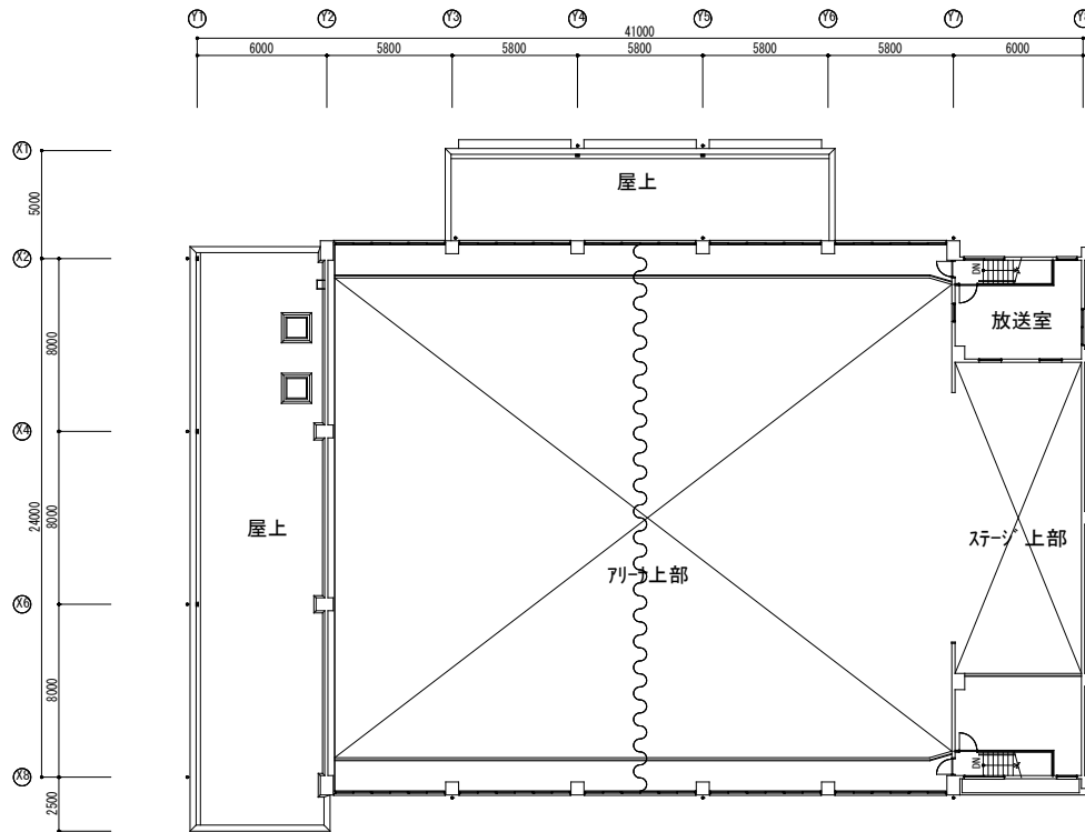
体育館 2 階平面図
