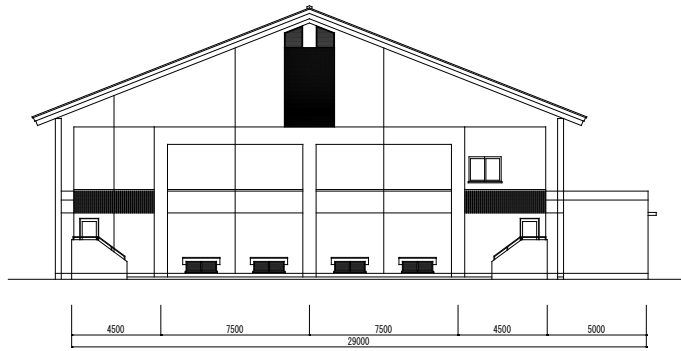
東側立面図
