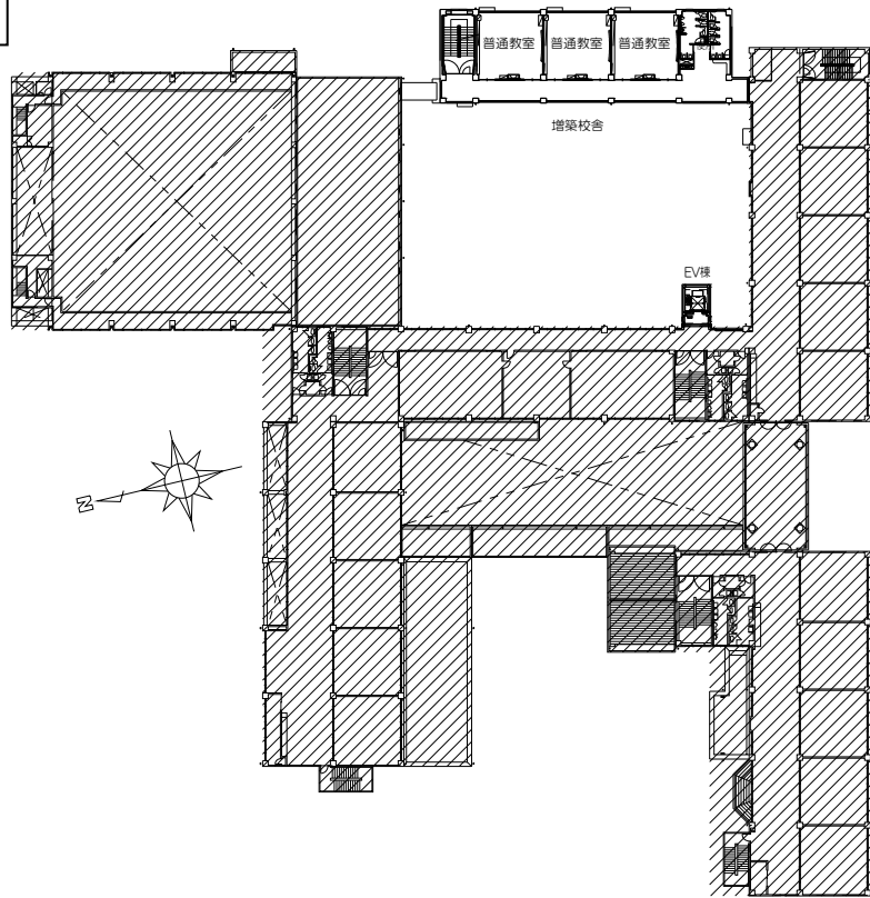
2 階平面図
