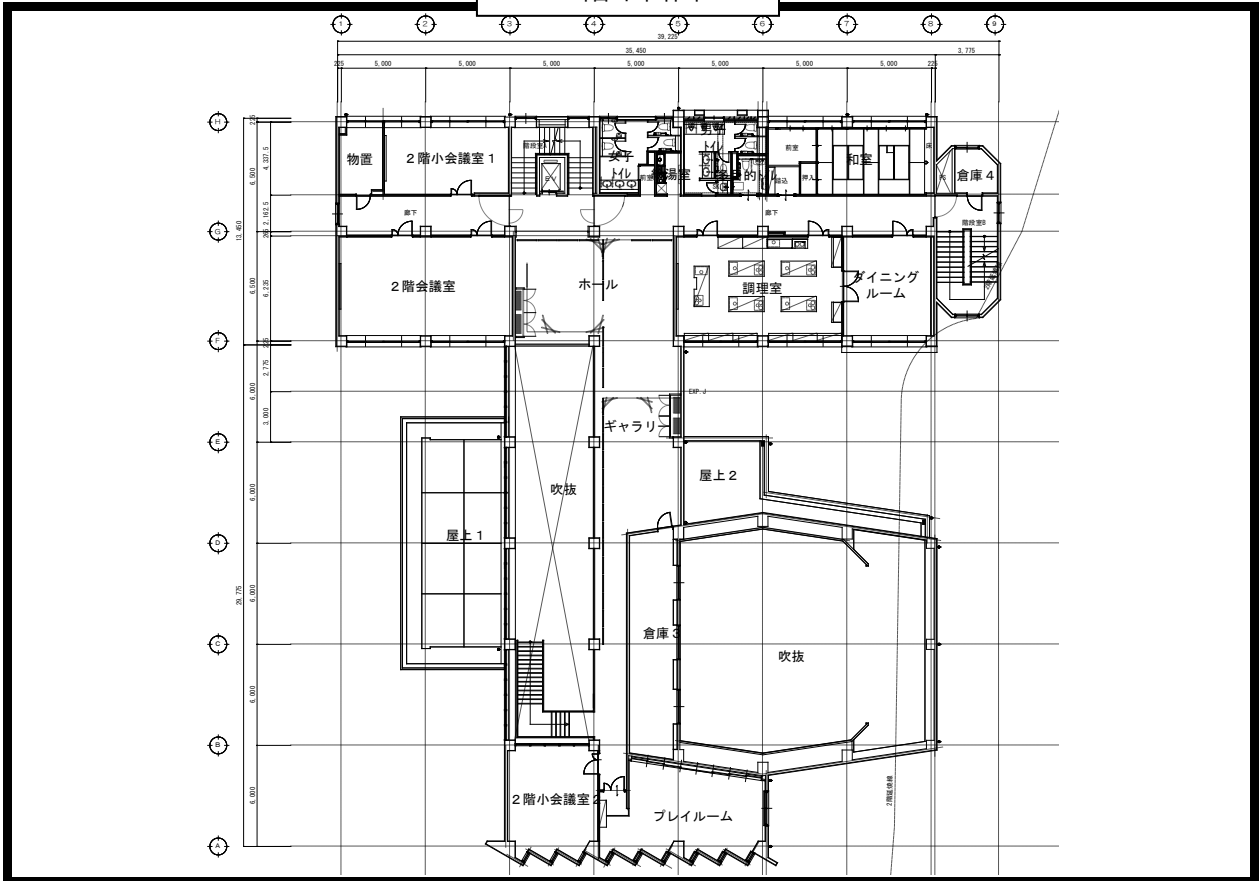
2階平面図
