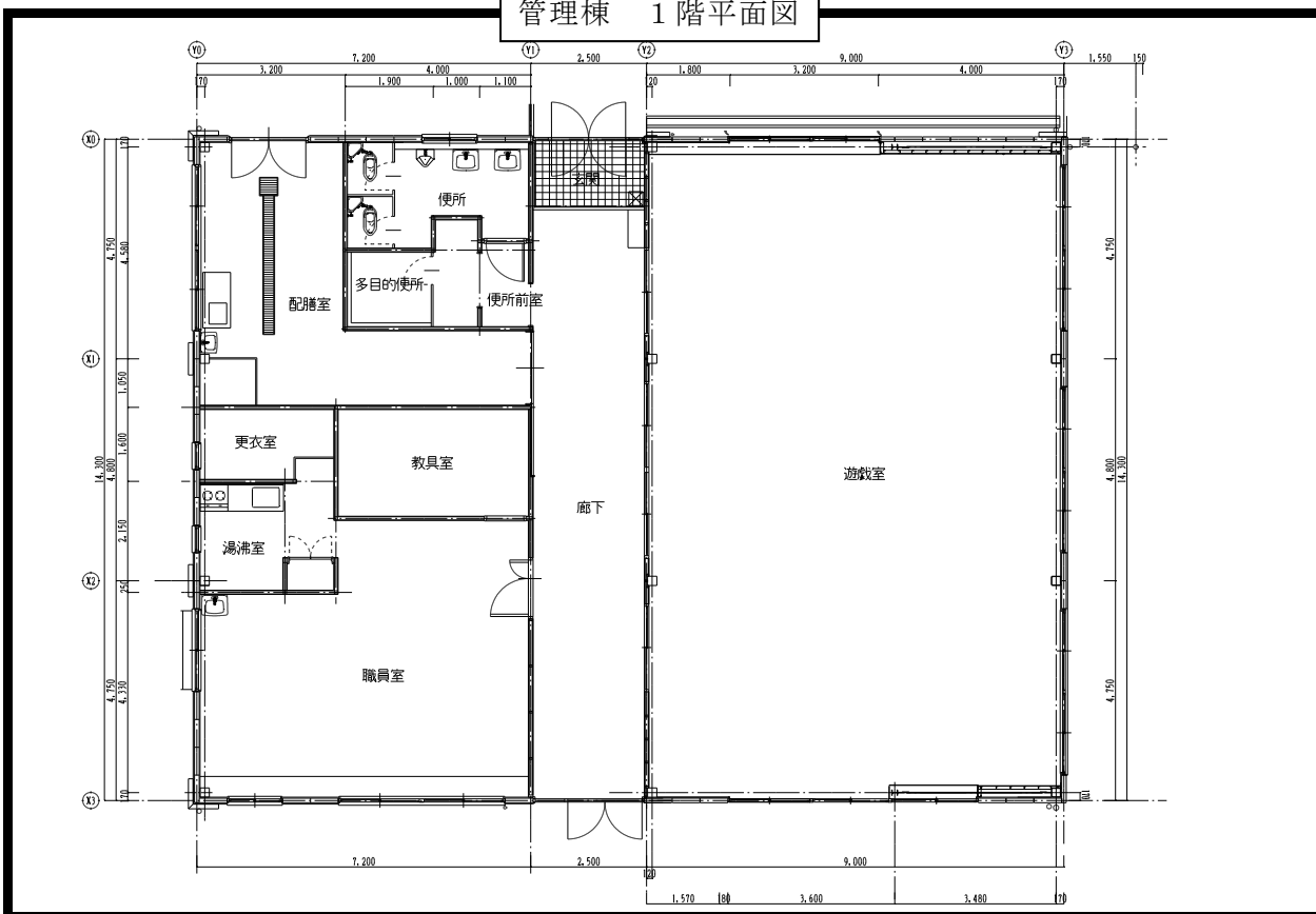
管理棟 1階平面図
