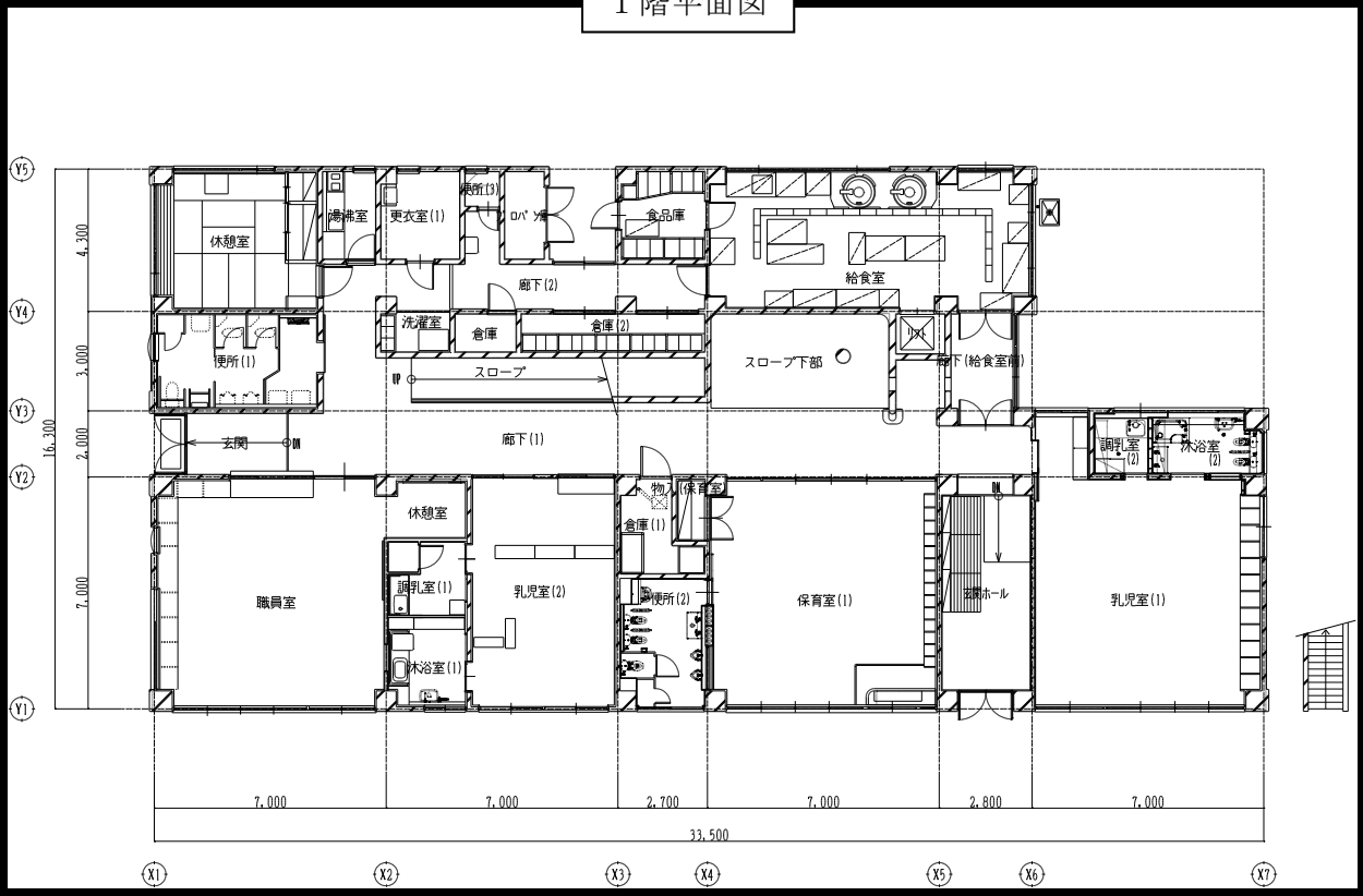
1階平面図
