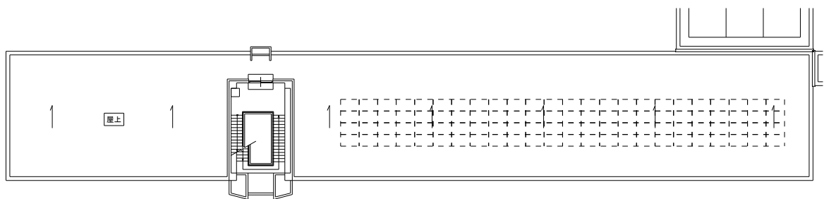
屋上平面図
