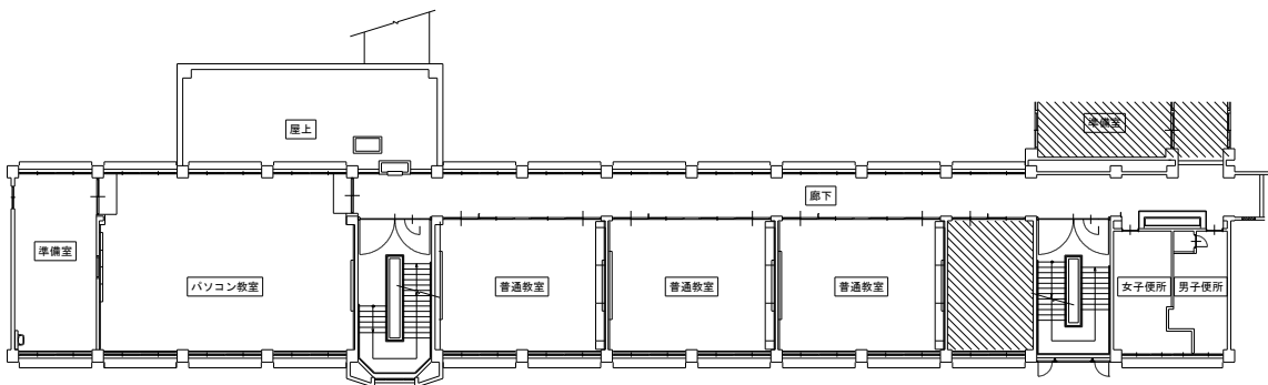
3階平面図
