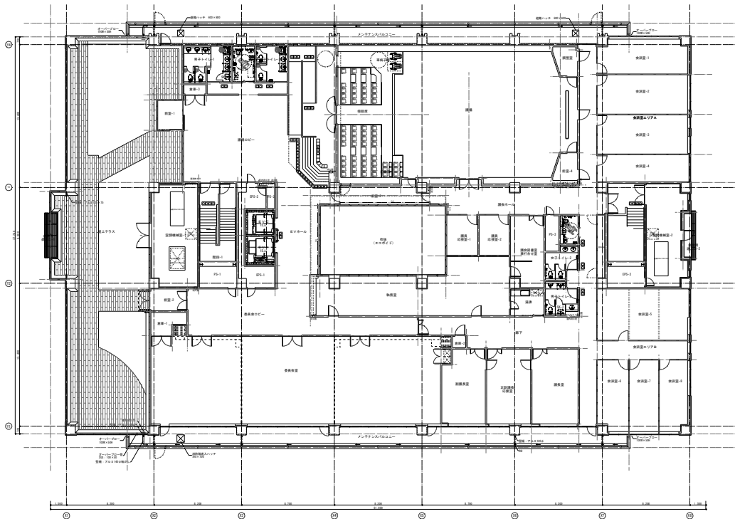
6階平面図
