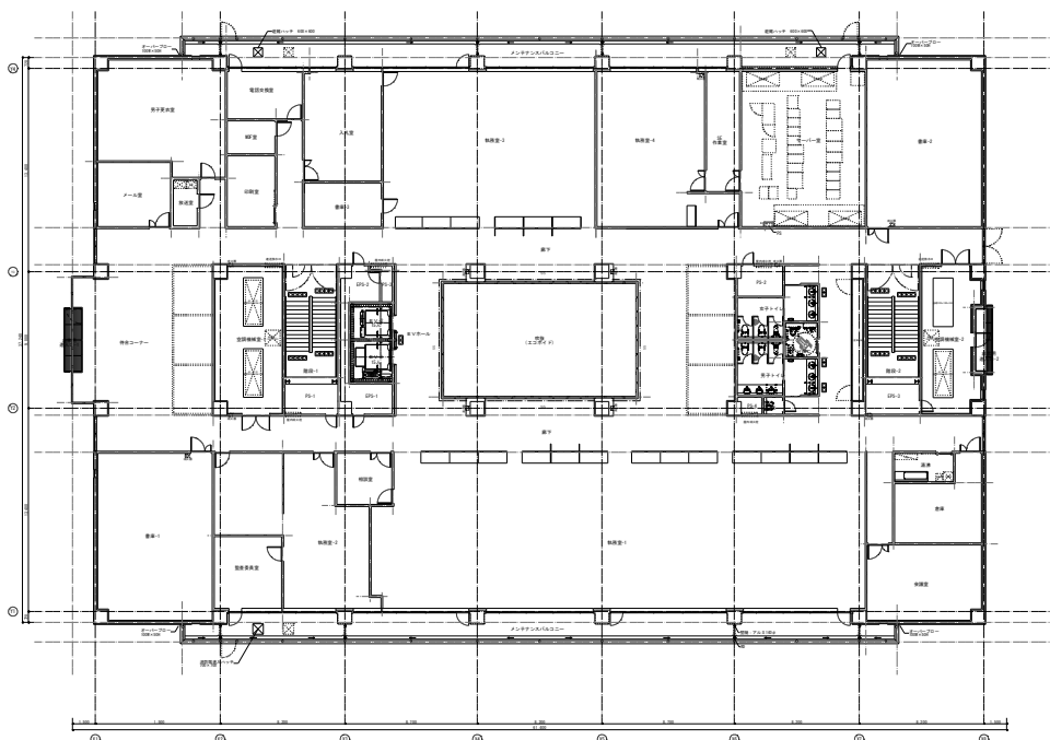
4階平面図
