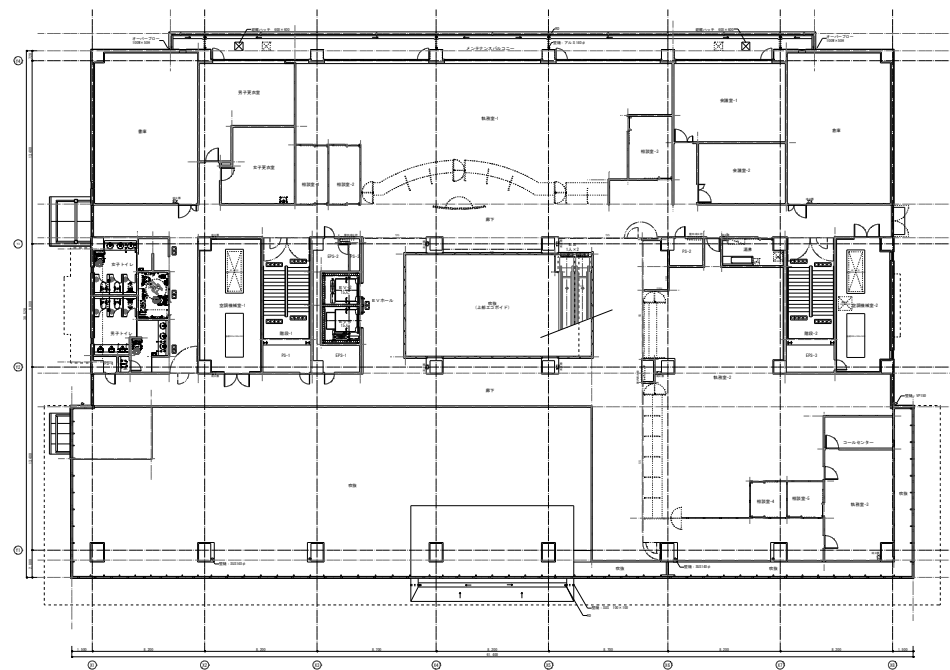
2階平面図
