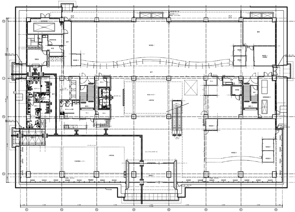
1階平面図
