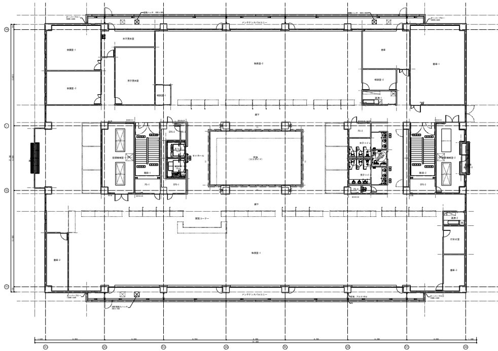
5階平面図
