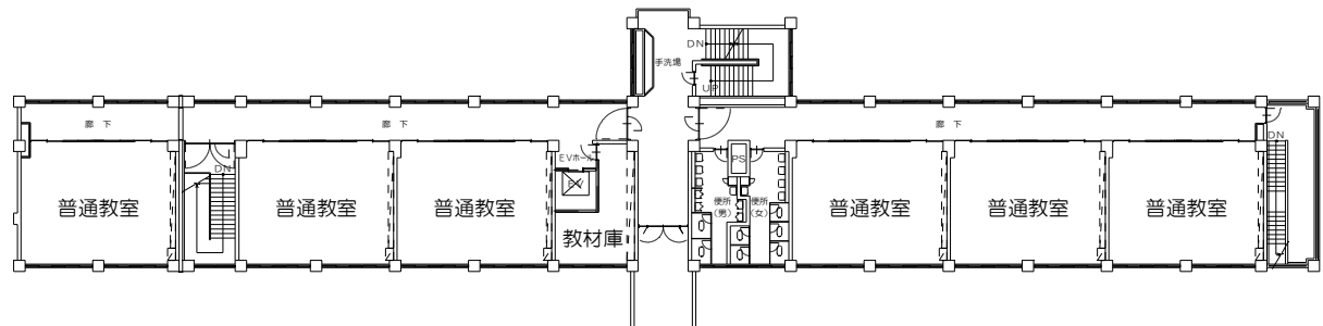
4階平面図 1/200
