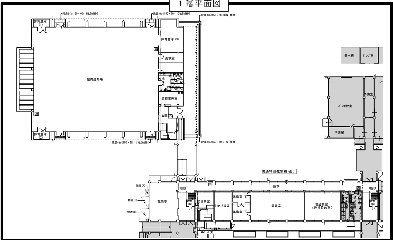
1階平面図
